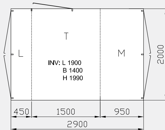
Frit dørmål b=1800 h=1900
