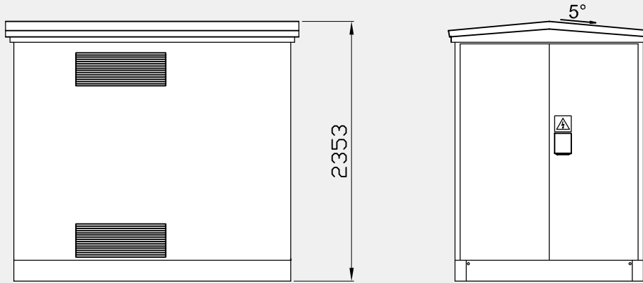
Frit dørmål b=1500 h=1900
