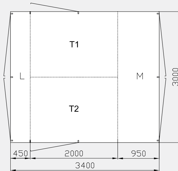
Frit dørmål b=2800 h=1900
