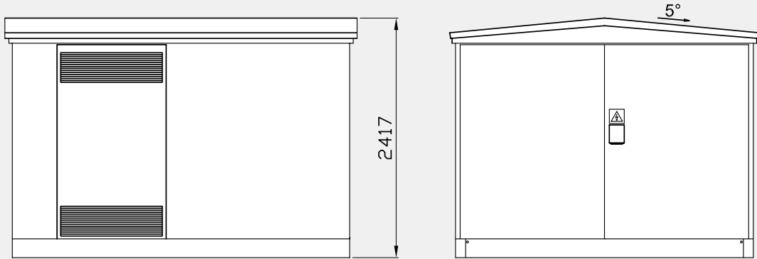
Frit dørmål b=2800 h=1900
