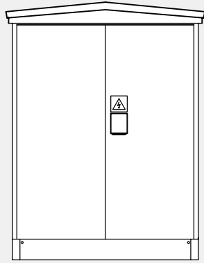
Frit dørmål b=1500 h=1900
