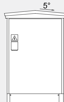
Frit dørmål b=1060 h=1600
