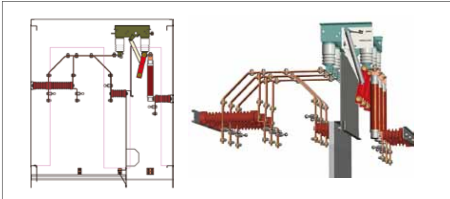
Eksempel på bestykning med mellemspændingsadskiller, m. sikringsholder, tre kabeltilslutninger, og anbringelse af afskærmningsplade
